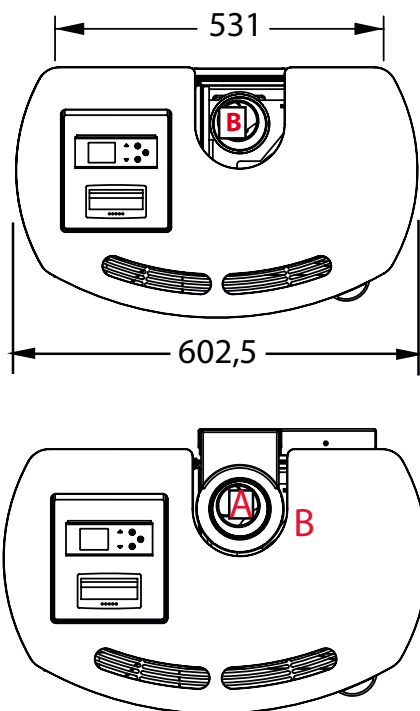
Vista dall'alto / Top view / Vista superior / Draufsicht
